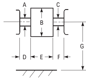
B & E...Max Cplg Dim D & F...Exposed Shaft
